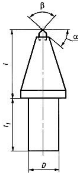
Рисунок 3 - Резец исполнения ТП
