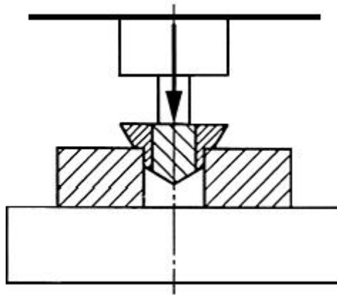
Рисунок А.2 - Схема определения прочности соединения армирующей вставки с державкой для резцов, армированных в закрытый паз цилиндрической вставкой
