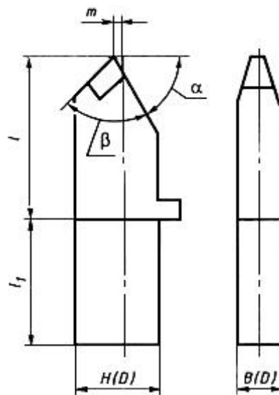
Рисунок 2 - Резец исполнения ТН
