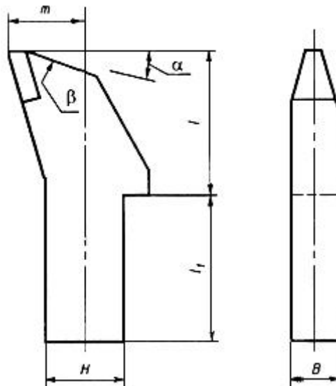
Рисунок 1 - Резец типа Р
